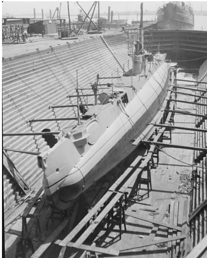
Submarino tipo “Holland” en construcción
